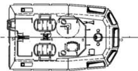
Topdeck
